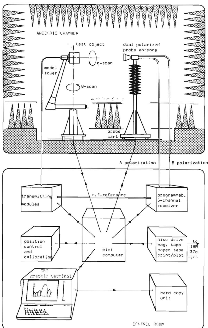
Fig. 1: Antennemeetfaciliteit ontwikkeld voor opdrachten van de ruimtevaartindustrie, TH Denemarken.
