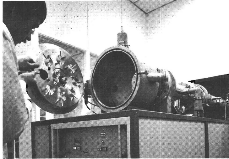
▲ De ionenimplantatie van de siliciumplakke gebeurt in de substraatkamer. In de dikke deur van deze machine kunnen totaal acht plakken gemonteerd worden (links op foto). De hoogspanningskamer ligt achter de rechter wand. Dit is te zien in het IC-atelier van de TH-Twente.
