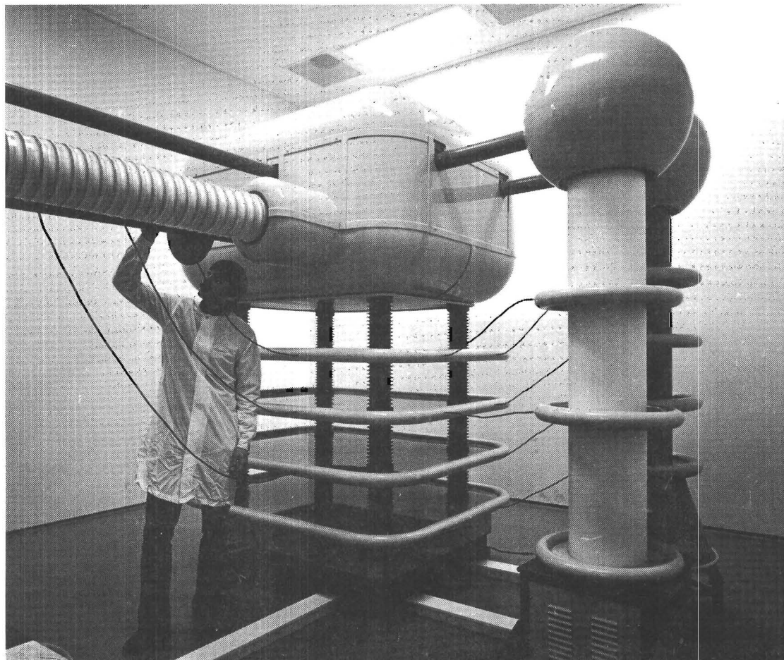
Dit is het hoogspanningsgedeelte van de ionenimplantatiemachine, zoals die in het IC-atelier van de TH-Twente staat opgesteld.
