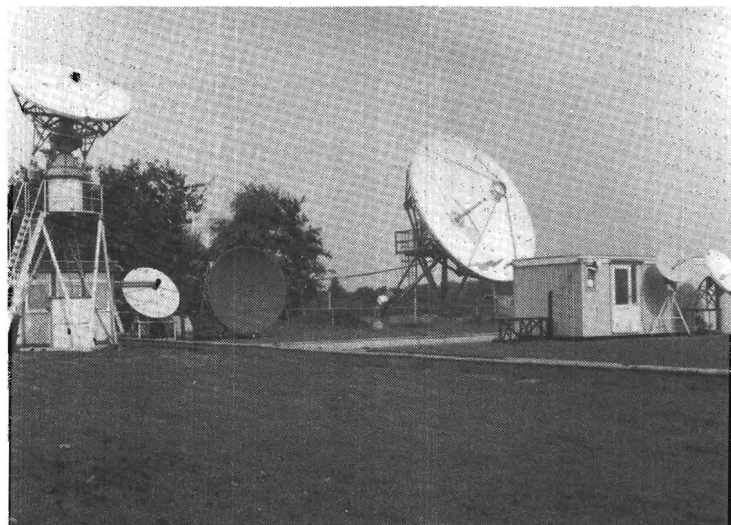
De geslaagde experimenten werden uitgevoerd met de acht meter parabool (grootste op foto), die in het antennepark op het THE-complex staat.
