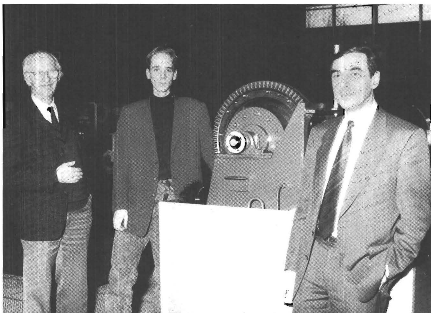
Van links naar rechts Peer Hezemans, Mark Peerdeman en Jeu Schouten bij een kroonwieltestopstelling. Foto: Hans van der Burg/RF
